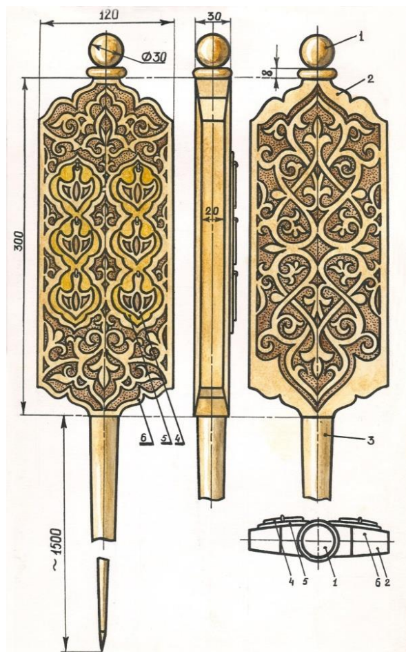
Сылдырмақ асатаяқтың сызбасы. Суретші Адамкулов Н.М.
