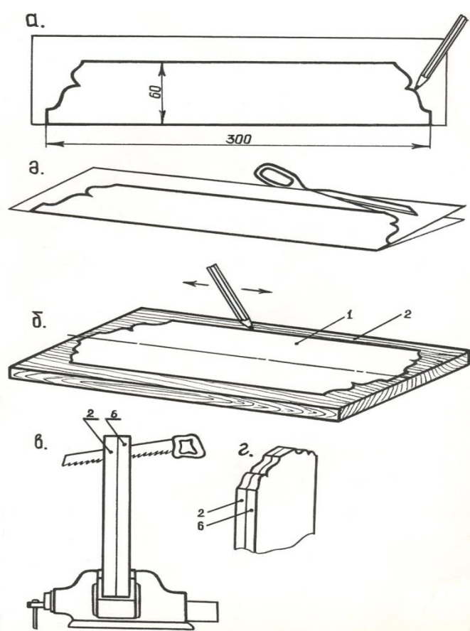
Асатаяқтың өлшемдері. а-б, қағазға түсірілген өлшемдері, в-ағашқа түсіру ережесі, г-өңдеу кезеңі. Суретші Адамқұлов Н.М.
